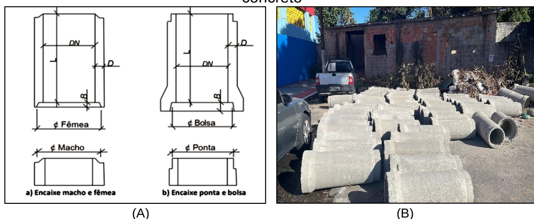
Figura 1 – (A) Corte de tubos encaixe ponta bolsa e macho-fêmea (B) Tubo de concreto
