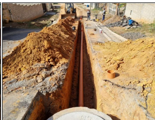
Figura 2 - Rede coletora de esgoto
