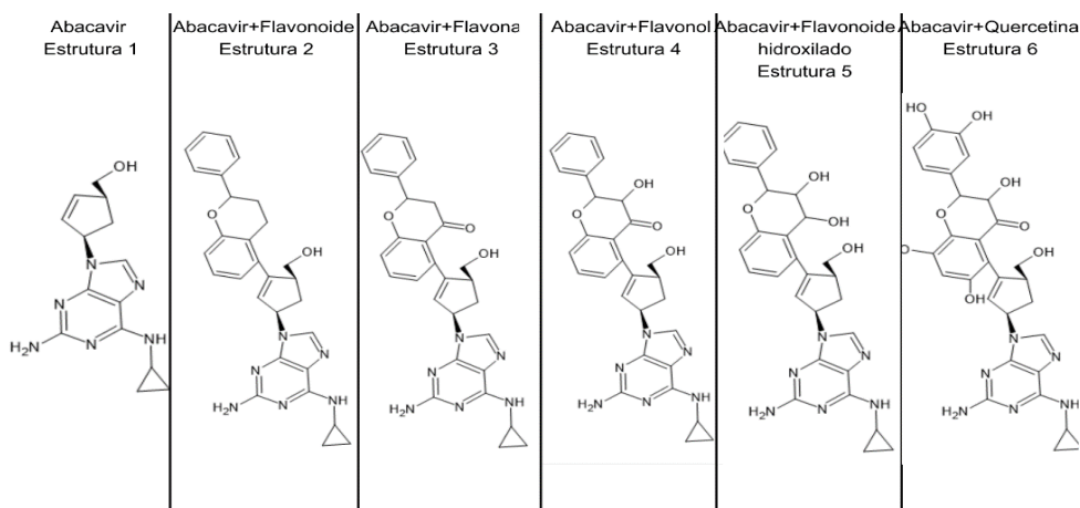
Figura 5 - Modificações do abacavir
