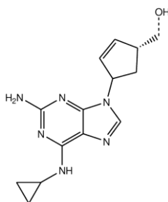
Figura 2 - Estrutura química do Abacavir
