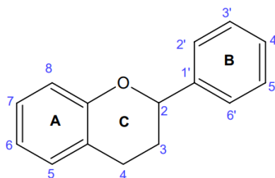
Figura 3 - Estrutura base dos flavonoides
