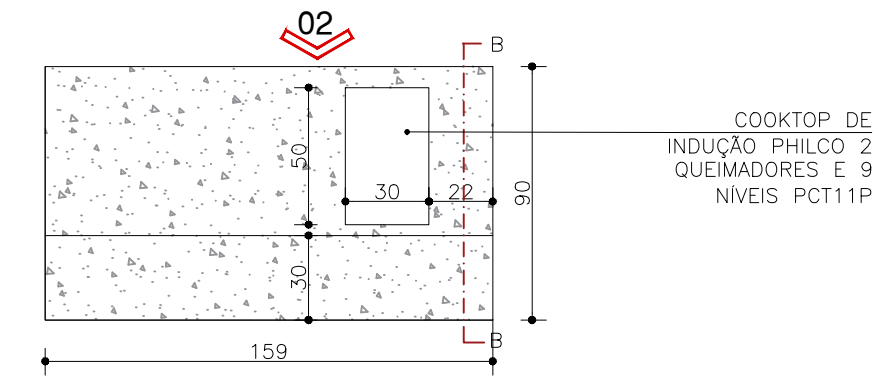
PLANTA BAIXA – COZINHA
