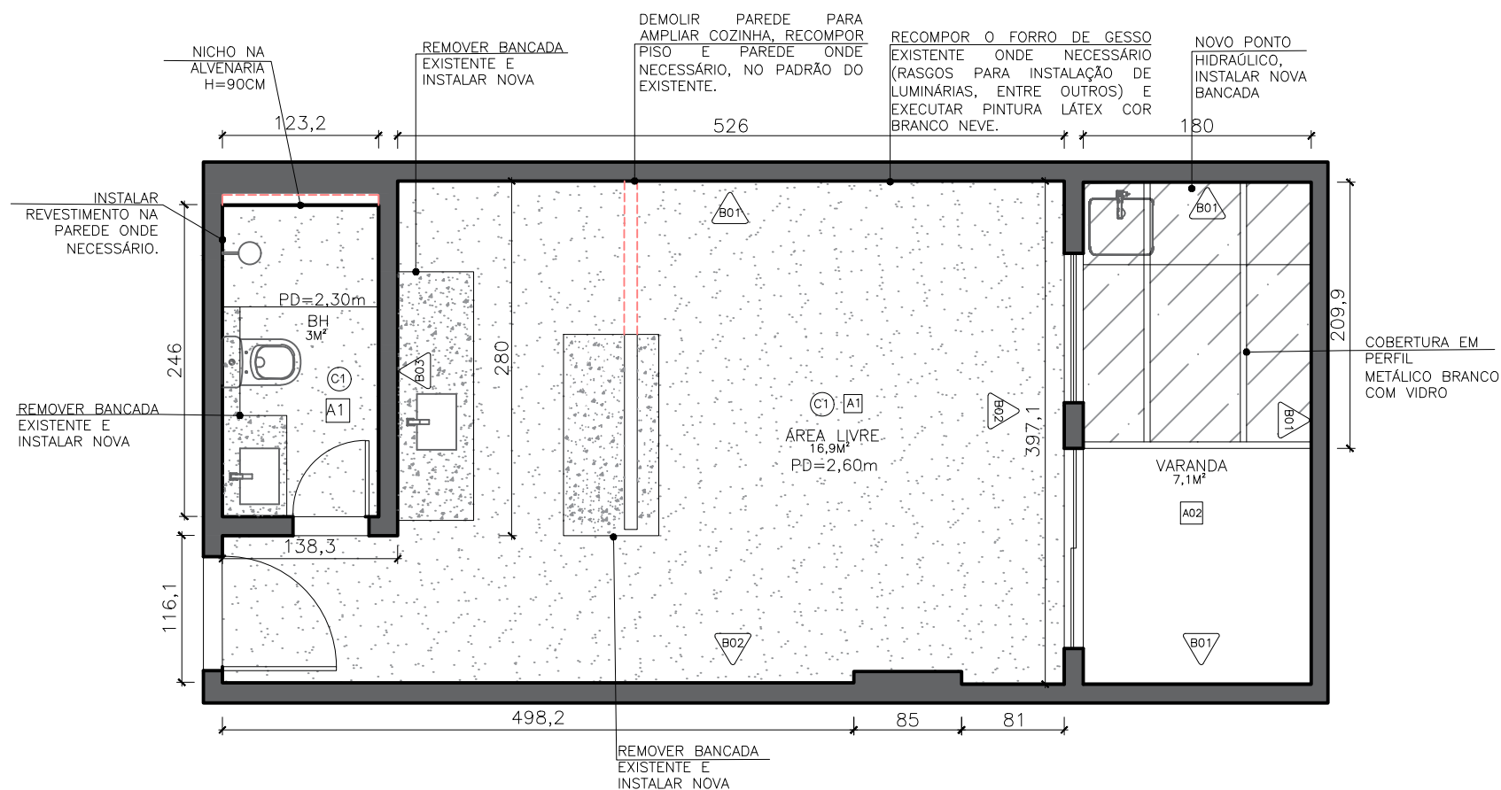
PLANTA REFORMA ESC: 1/50
