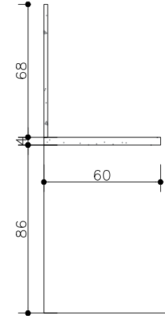
CORTE AA ESCALA 1/25
