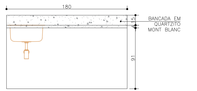
VISTA 03 ESCALA 1/25
