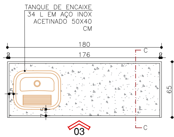
PLANTA BAIXA – ÁREA SERVIÇO
