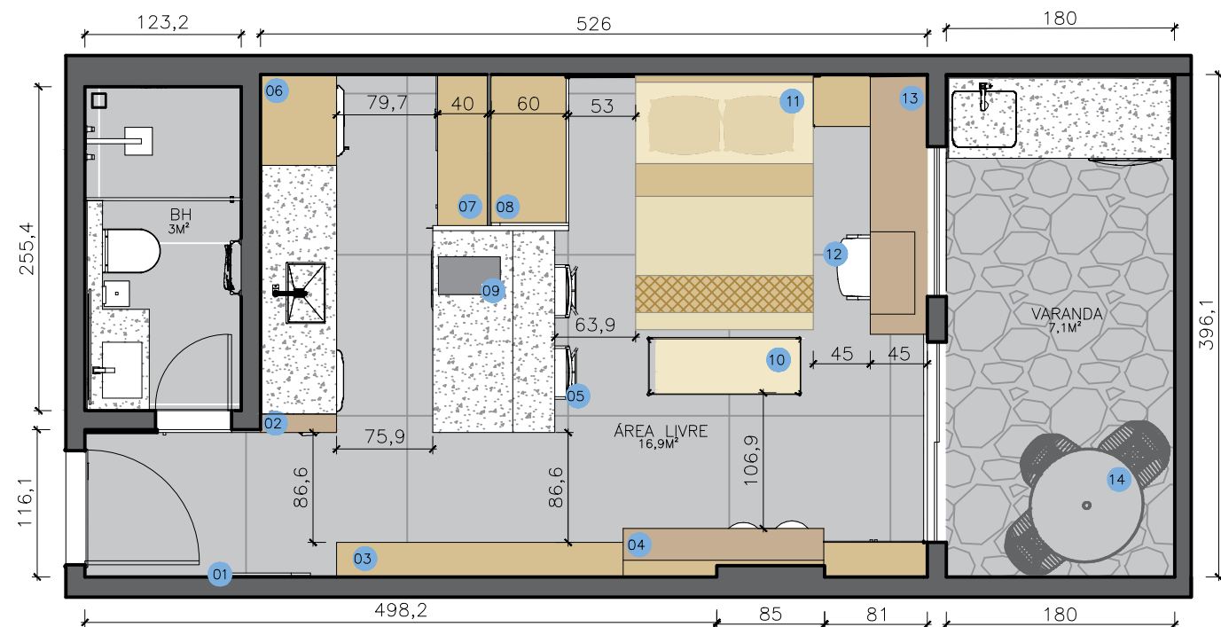
PLANTA LAYOUT ESC: 1/50
