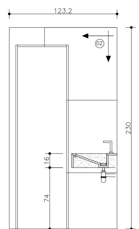
VISTA 04 – BH SUITE ESCALA 1/25
