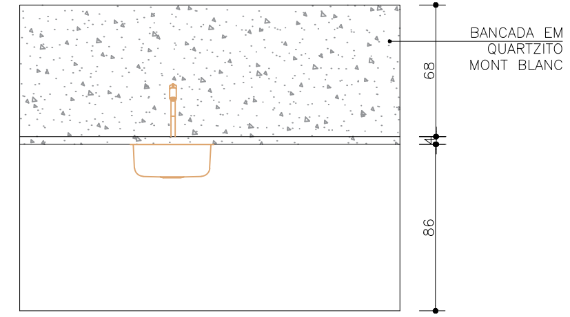
VISTA 01 ESCALA 1/25
