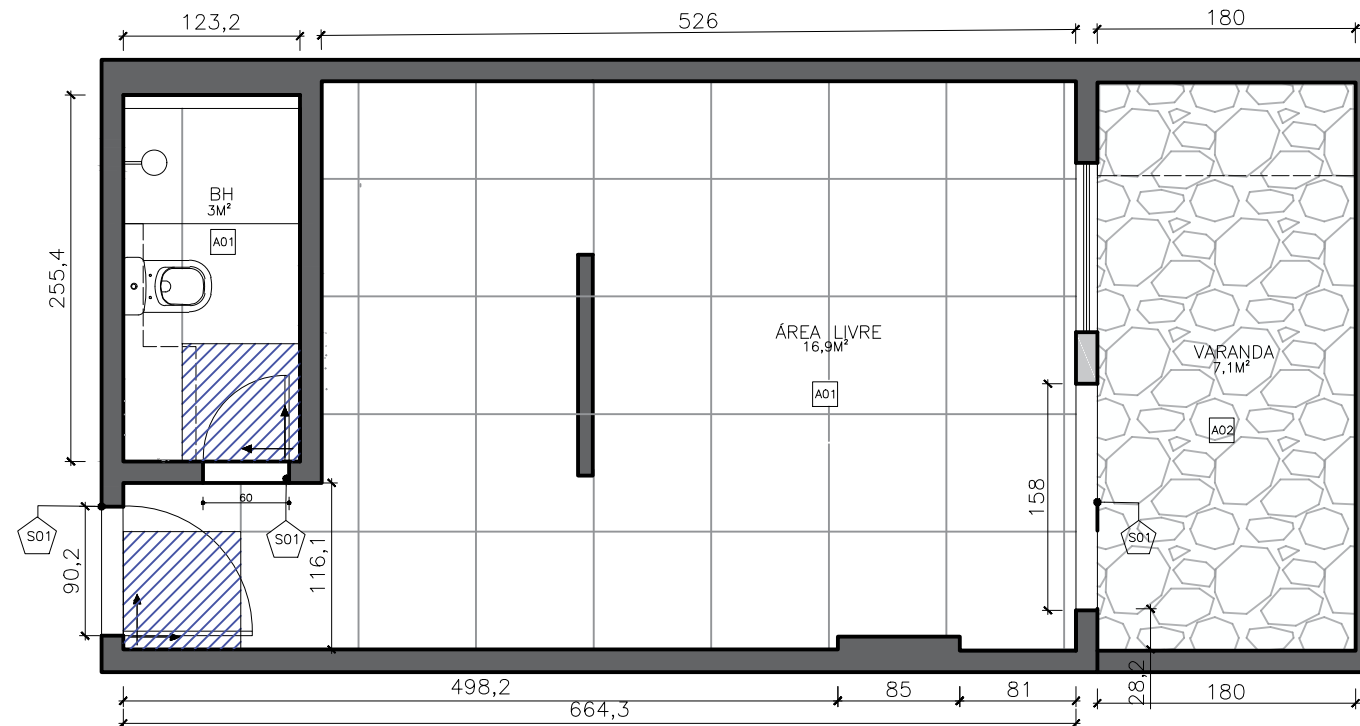
PLANTA PAGINAÇÃO DE PISO ESC: 1/50
