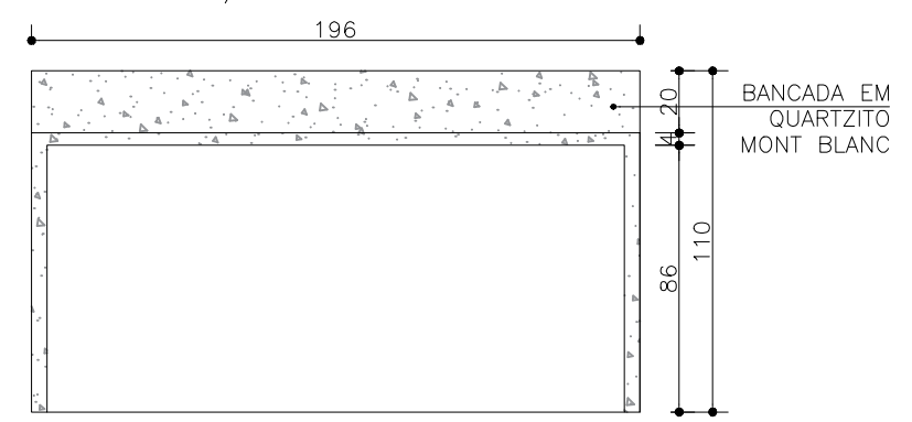
VISTA 02 ESCALA 1/25
