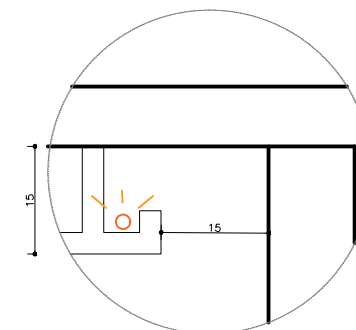
SANCA ILUMINAÇÃO ESC: 1/5
