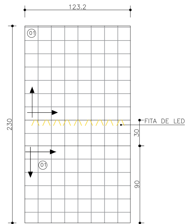
VISTA 02 – BH SUITE ESCALA 1/25
