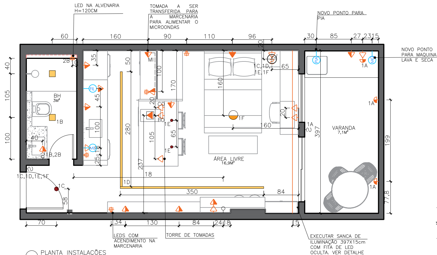
PLANTA INSTALAÇÕES ESC: 1/50
