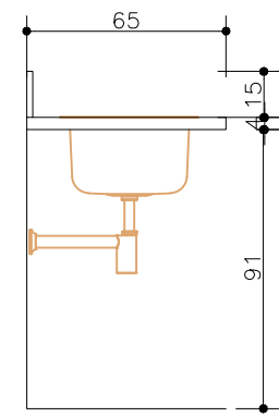
CORTE CC ESCALA 1/25
