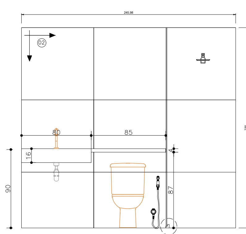
VISTA 01 – BH SUITE ESCALA 1/25
